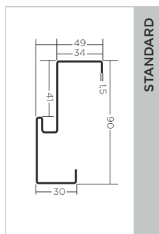
ościeżnica PU56
