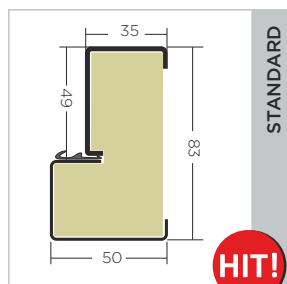
ościeżnica Termo ODS68
