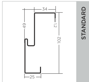
ościeżnica PU68
