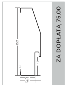
ościeżnica PD56/150
